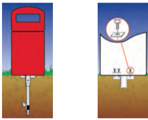
Afvalbak geïnstalleerd met Ground-Lock-systeem. Binnenaanzicht van de afvalbak met de boutbevestiging aan het Ground-Lock-systeem.
