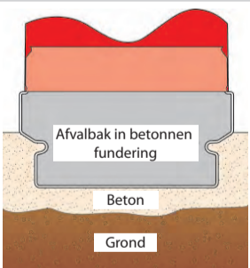
H) Betonneren
